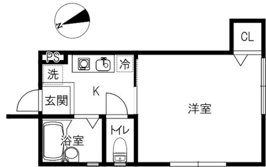
Room layout 洋7 K (専有面積: 21.09㎡)
